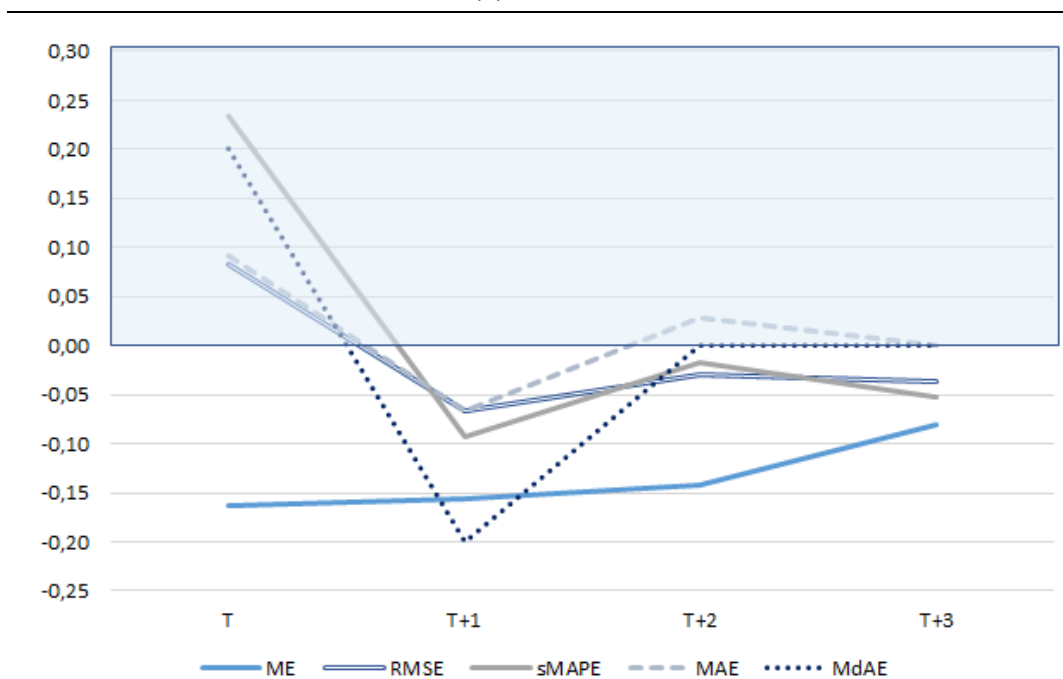
Fig. 6 – Differenza tra le diagnostiche previsionali calcolate con dati ex post rispetto a quelle con dati preliminari (1)
