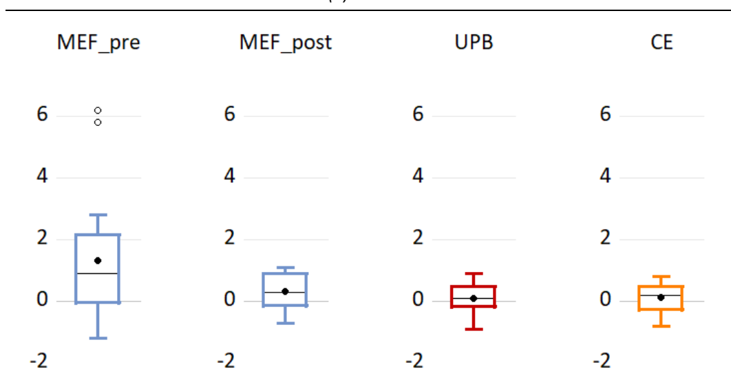
Fig. 5 – Boxplot degli errori di previsione per l'anno T+1 (1)
